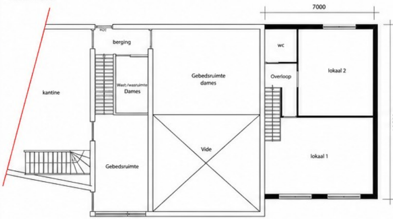
BESTAANDE SITUATIE VERDIEPING (MAATVOERING)
