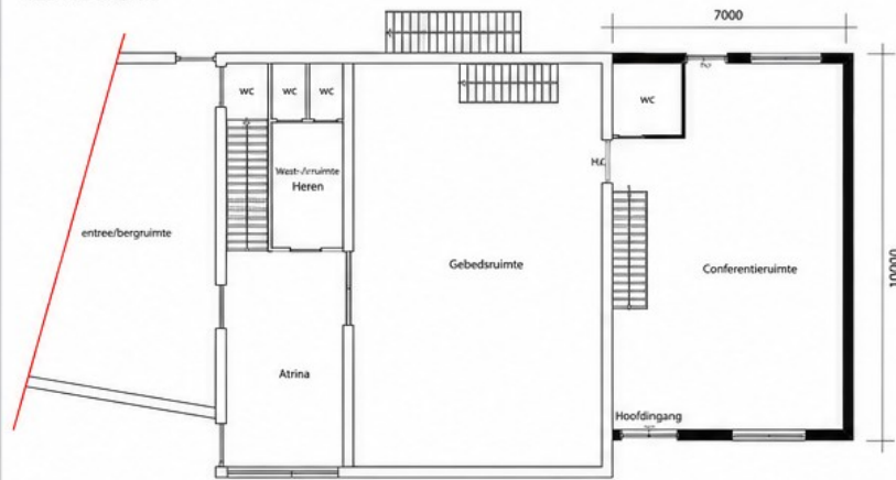
BESTAANDE SITUATIE BEGANE GROND (MAATVOERING)
