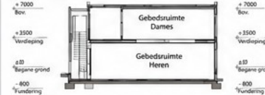
DOORSNEDE A-A
